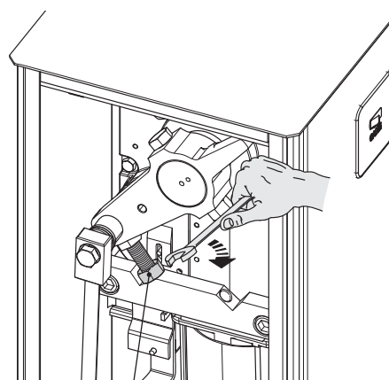
Контргайка
